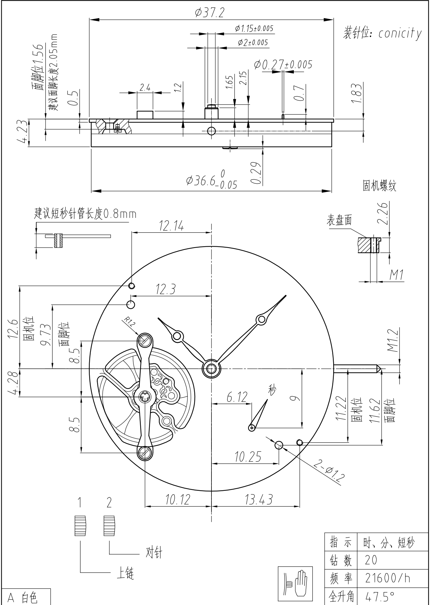
HZ93A0A 短秒3针 5字位小秒 (摆轮位镂空)
